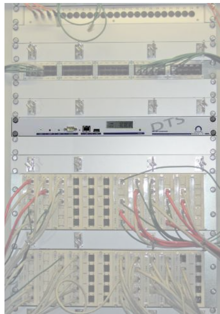
Appareil DTS, monté dans un rack IT de 19"
